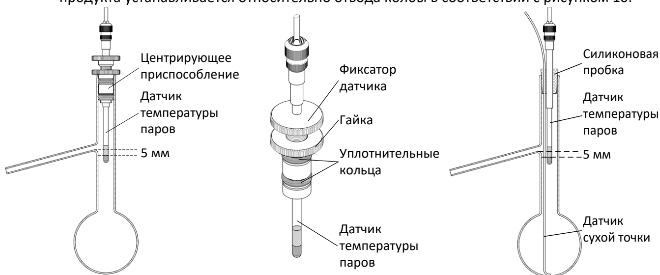
Рисунок 10 – Установка датчика температуры паров
