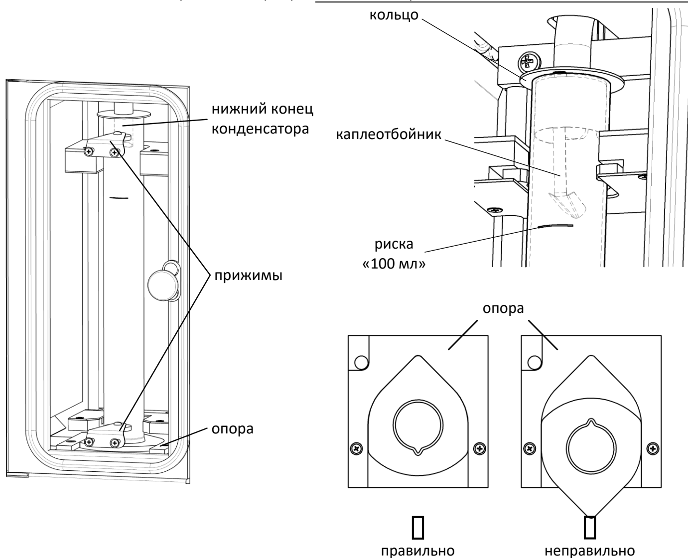
Рисунок 11 – Установка мерного цилиндра в приёмник
