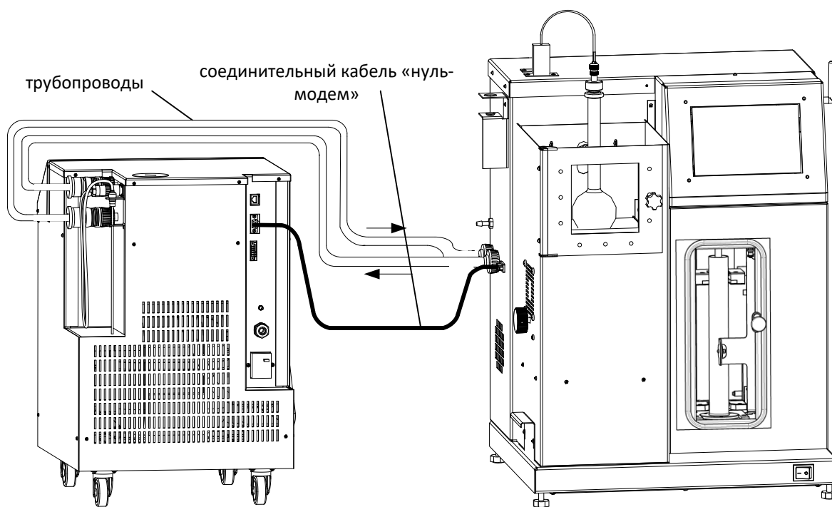
Рисунок 4 – Подключение к термокриостату ТКП-10
