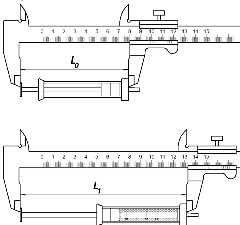
Рисунок Г1.1 – Измерение размеров шприца
