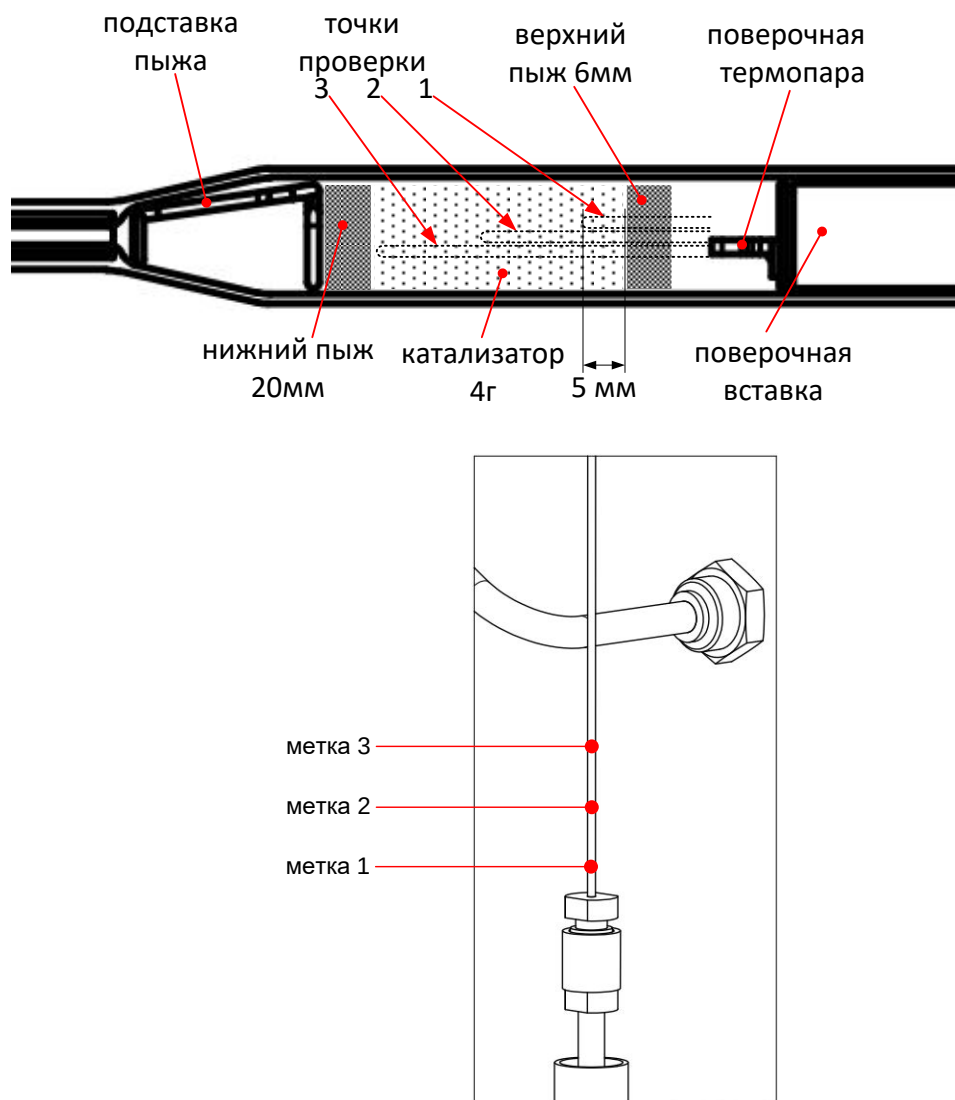
Рисунок А1.1 – Проверка температуры реактора
