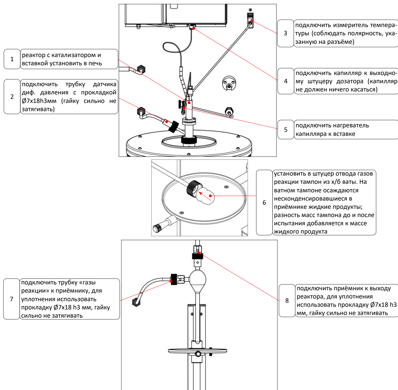
Рисунок 14 – Подключение реактора и приемника
