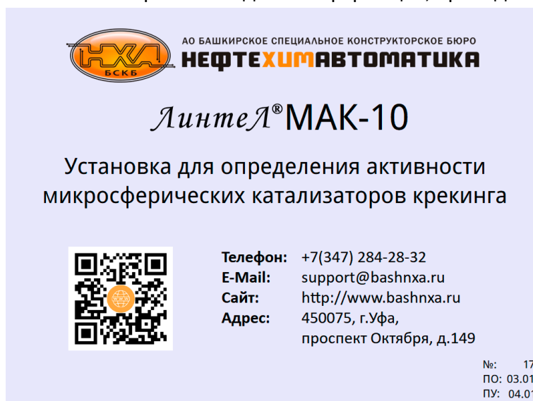
Рисунок 5 – Окно заставки
