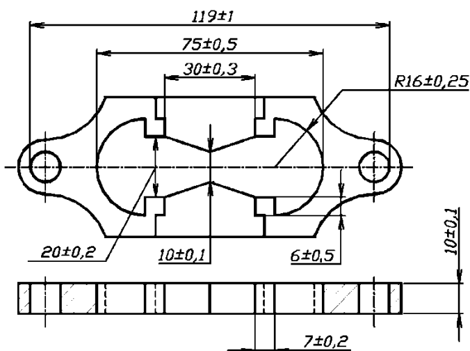
Размеры формы тип 1 АИФ 6.434.013-03
