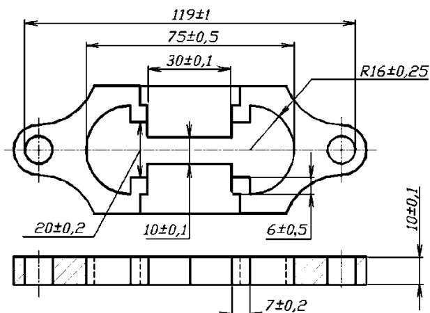
Рисунок 3 – Основные размеры формы в сборе для ASTM D 6084
