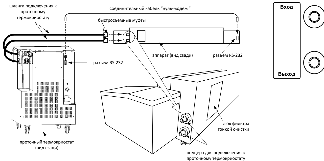
Рисунок 5 – Подключение к ТКП-10
