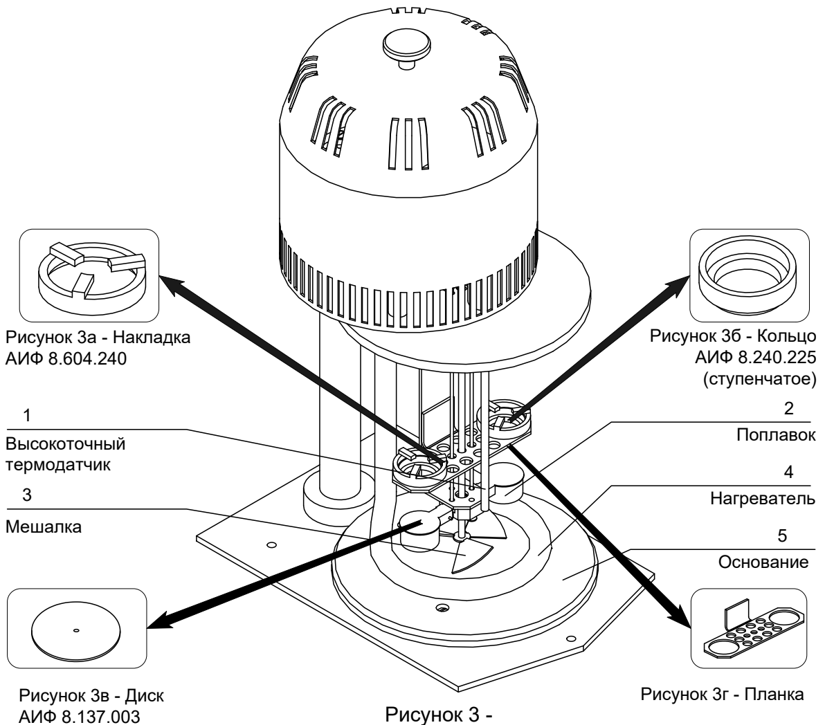
Рисунок 3 – Технологический блок
